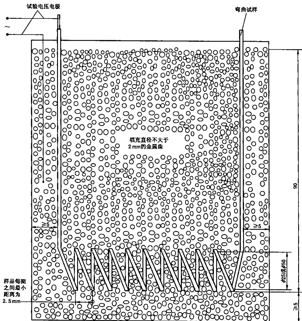
图 3a 击穿电压试验用试样
